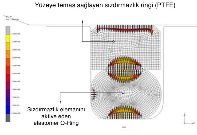
K17 SEA basınçsız durumda temas gerilimi
