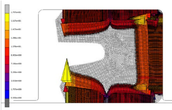
XT200®-050/1 200 bar basınç altında SEA analizi S akma boşluğu: 0.4 mm
