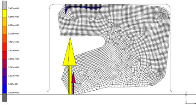
Resim 3.10 XT200 temas gerilimi (montaj durumu-basınçsız)
