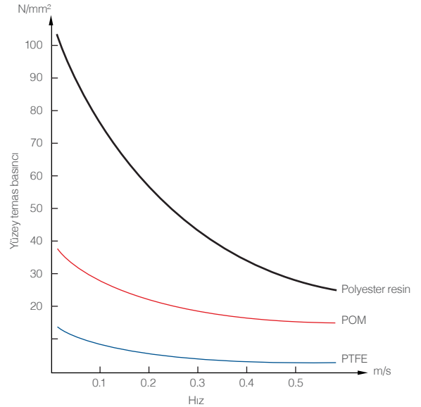
60 °C'de yataklama elemanları yüzey teması - hız grafiği
