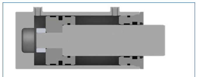
Çift etkili silindir
