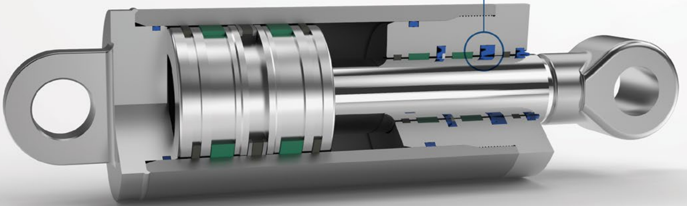
Hidrolik Boğaz Sızdırmazlık Elemanları
